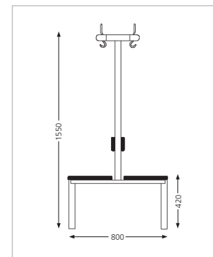
Doppelseitige Sitzbank mit Hakenleiste und Rückenlehne
